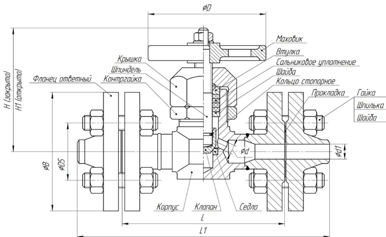
Основные параметры клапанов
